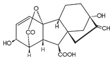
(2) GA_3 (gibberellic acid)
