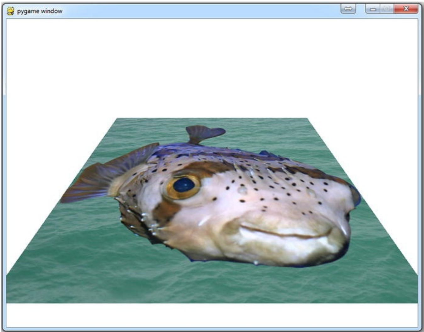
Figure 11-2. opengltext.py
