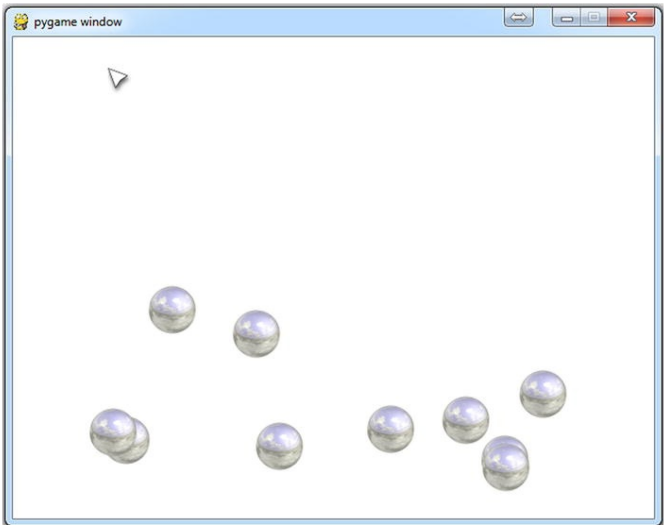
Figure 10-5. bouncesound.py
